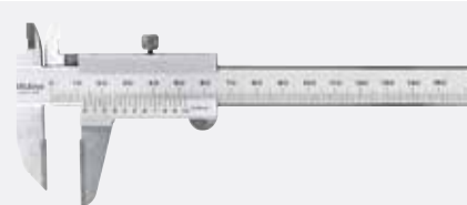
tip trasare cu fălci din carbură 536-221 | 536-222
